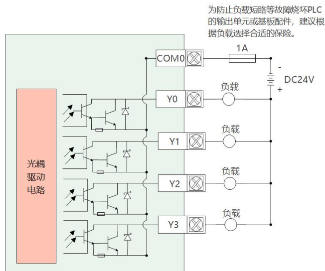
图 3-3 普通晶体管输出接线
