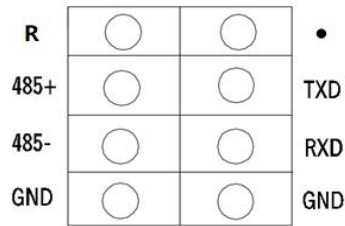
图 6-2 RS485 & RS232通信端口示意
