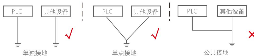
图 1-1 接地类型
